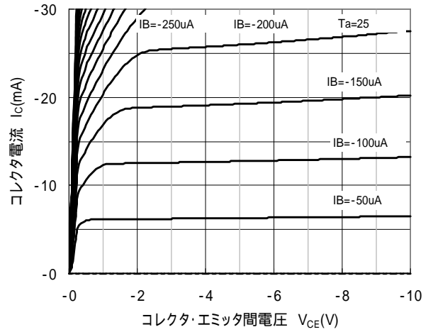
エミッタ接地出力特性 (1)
