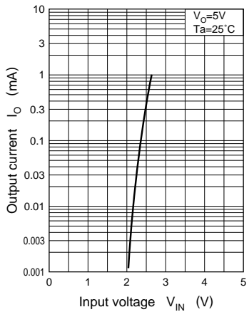
I_O - V_{IN}
