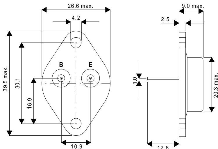
TO3 Package.
