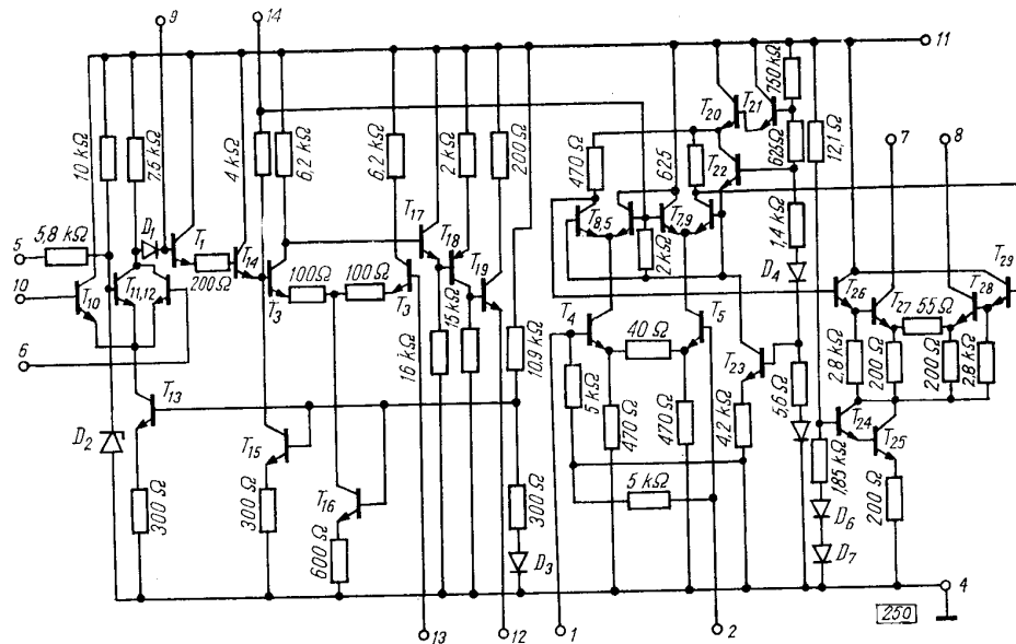
Schemat elektryczny
