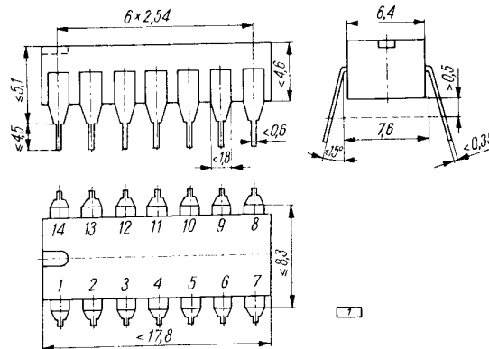
UKŁAD SCALONY W OBUDOWIE PŁASTYKOWEJ TYPU CE70 (TO-116)
