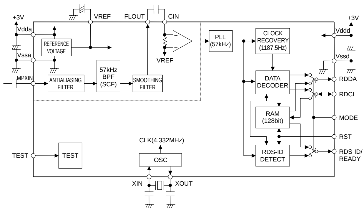
ブロック図
