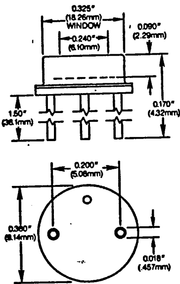
TO-5
