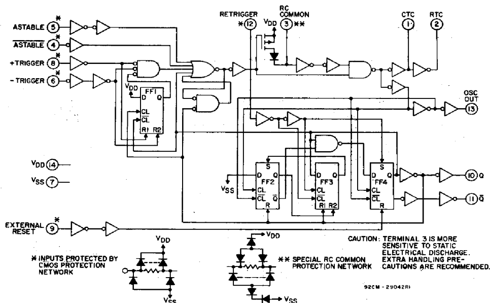
Fig. 2—CD4047B logic diagram.
