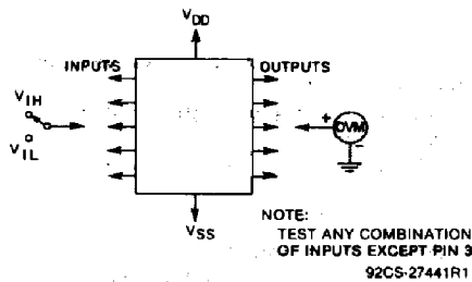
Fig. 30—Input-voltage test circuit.
