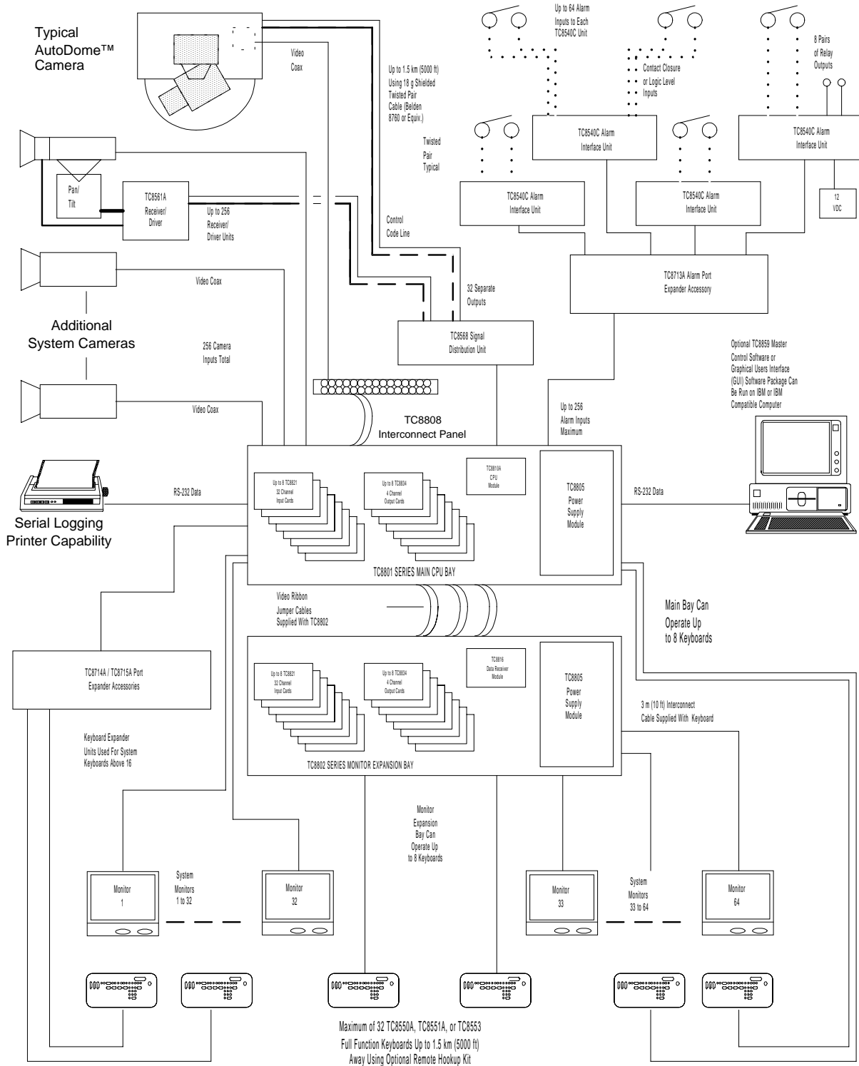
Configuración de capacidad completa TC8800
