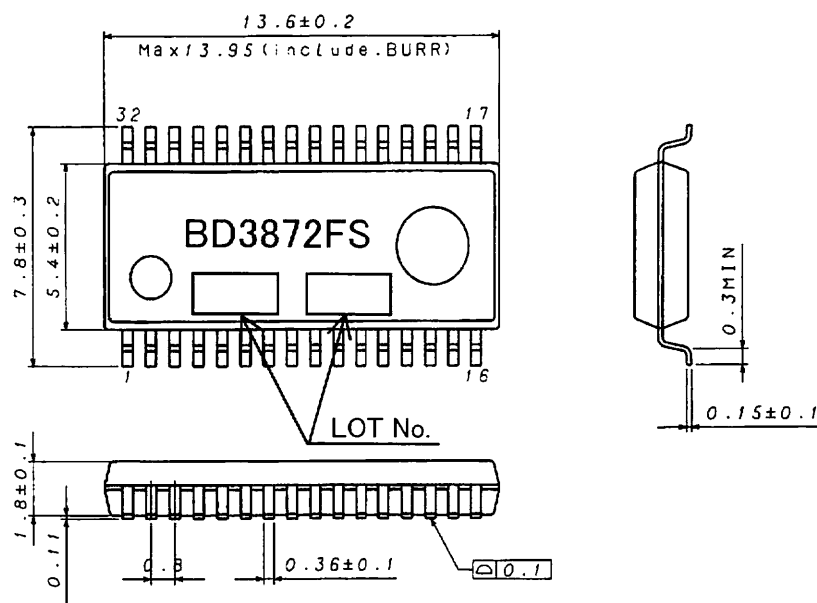
SSOP-A32(Unit:mm)
