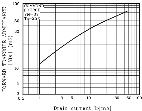
Fig.5 |Y_{fs}| - I_D
