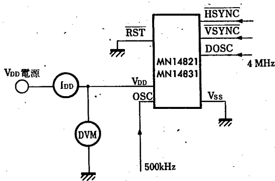
Fig. 3 電源電流(I DD )測定回路
