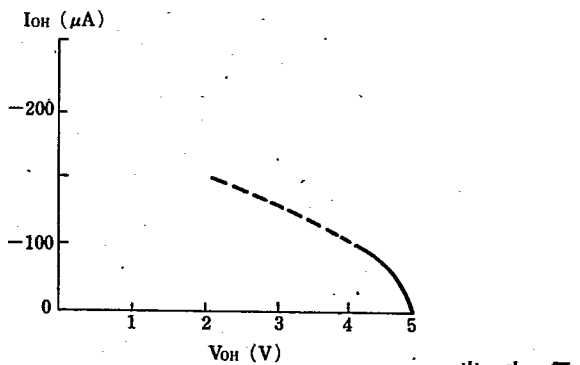
出力電流
