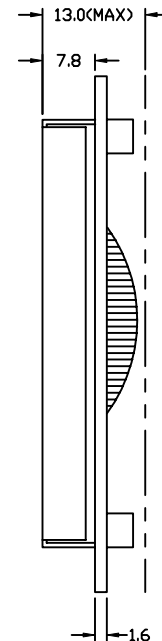
DETAIL: A
