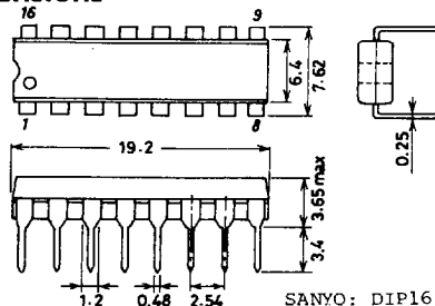
SANYO: DIP16
