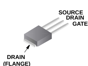
HUFA76629D3
