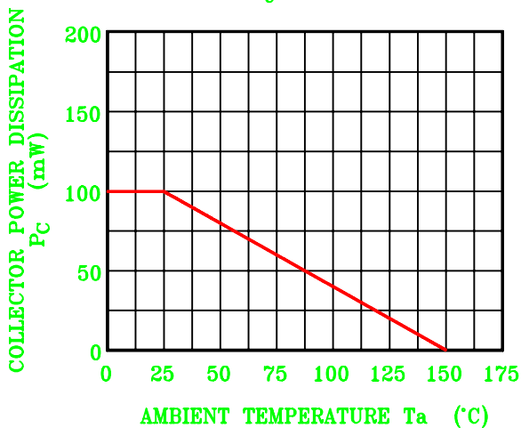
P_C - T_a
