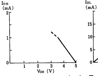
出力電流
