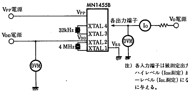
測定回路
