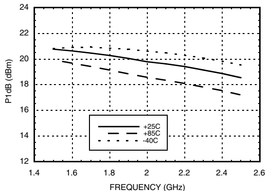
Output P1dB*
