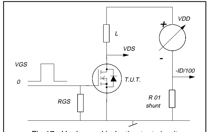
Fig.17. Unclamped inductive test circuit. E_{AS} = 0.5 \cdot L I_D^2 \cdot V_{(BR)DSS} / (V_{(BR)DSS} - V_{DD})
