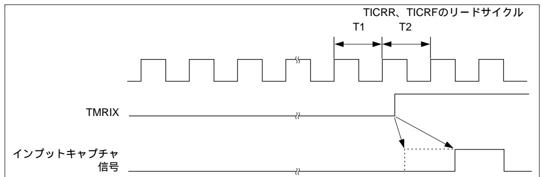
図 12.10 インพุットキャプチャ信号タイミング
