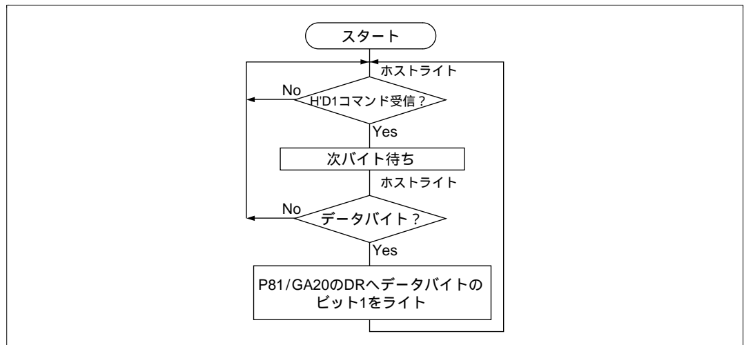
図 18.2 GA20 出力
