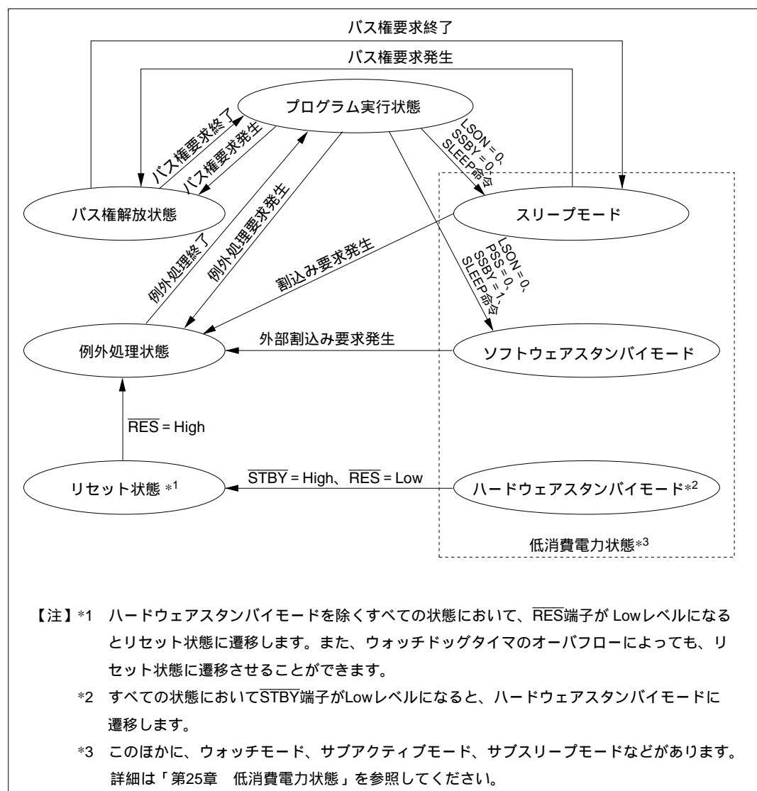
図 2.15 状態遷移図
