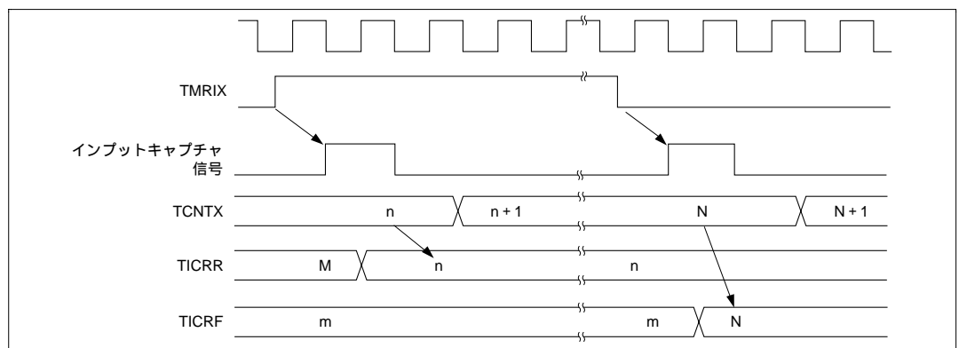
図 12.9 インพุットキャプチャ動作タイミング
