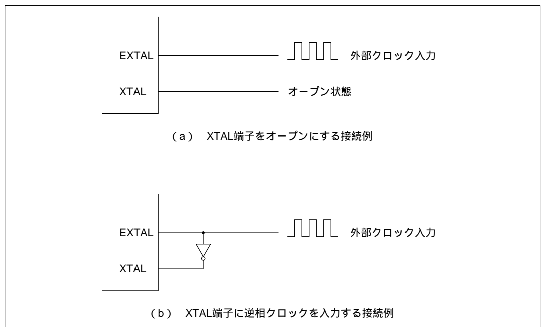
図 24.5 外部クロックの接続例
