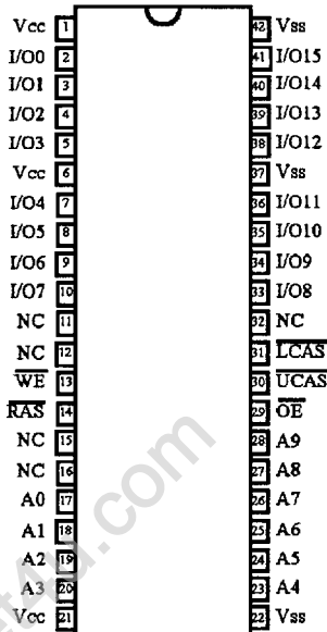
42 SOJ
