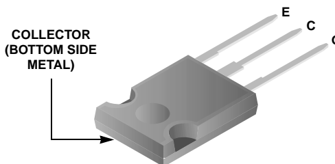
JEDEC STYLE TO-247
