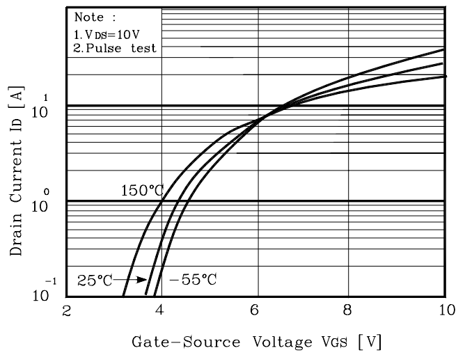
Fig. 2 I_D - V_{GS}
