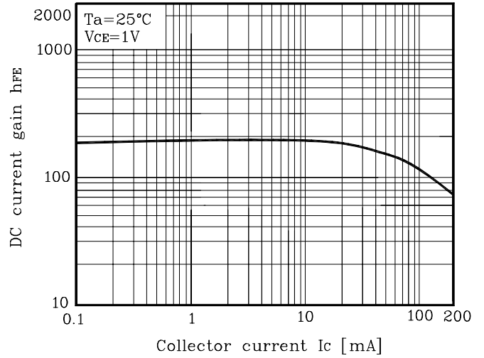
Fig. 2 h_{FE} - I_C
