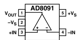
SOT23-5 (RT-5)
