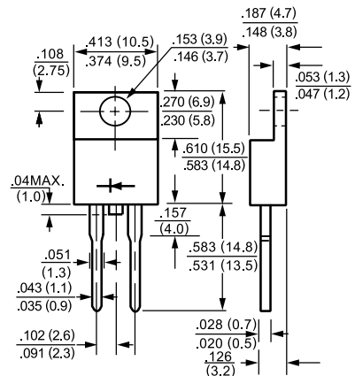
TO-220A
