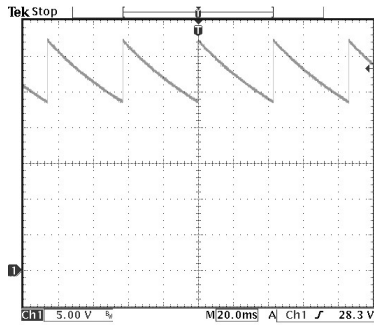
OVP Waveform
