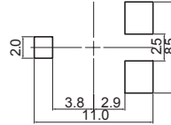
LAND PATTERNS (mm) 推奨ランド寸法
