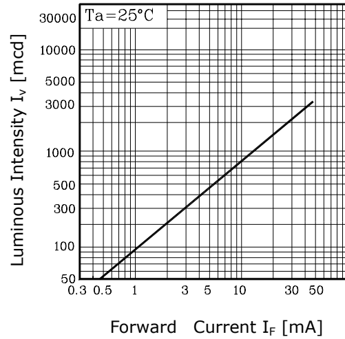
Fig. 2 I_V - I_F
