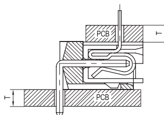
PCB ASS'Y
