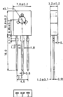
図1 JEDEC:TO-126M
