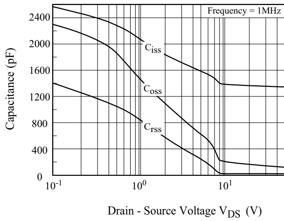
C - V_{DS}
