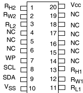
20 Pin TSSOP
