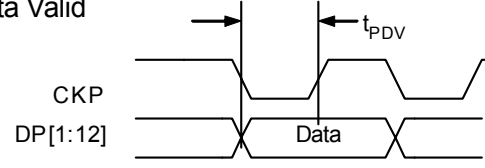
Data Valid
