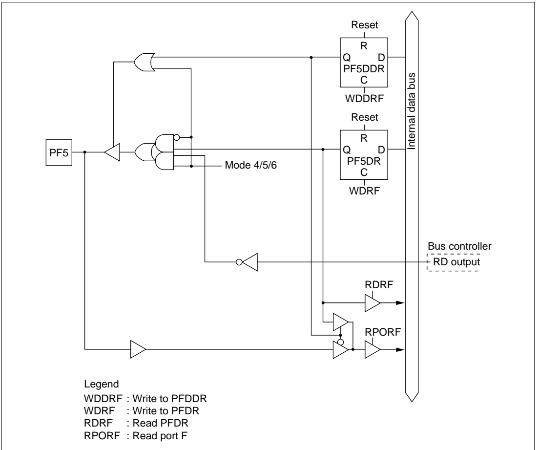
Figure C-10 (d) Port F Block Diagram (Pin PF5)
