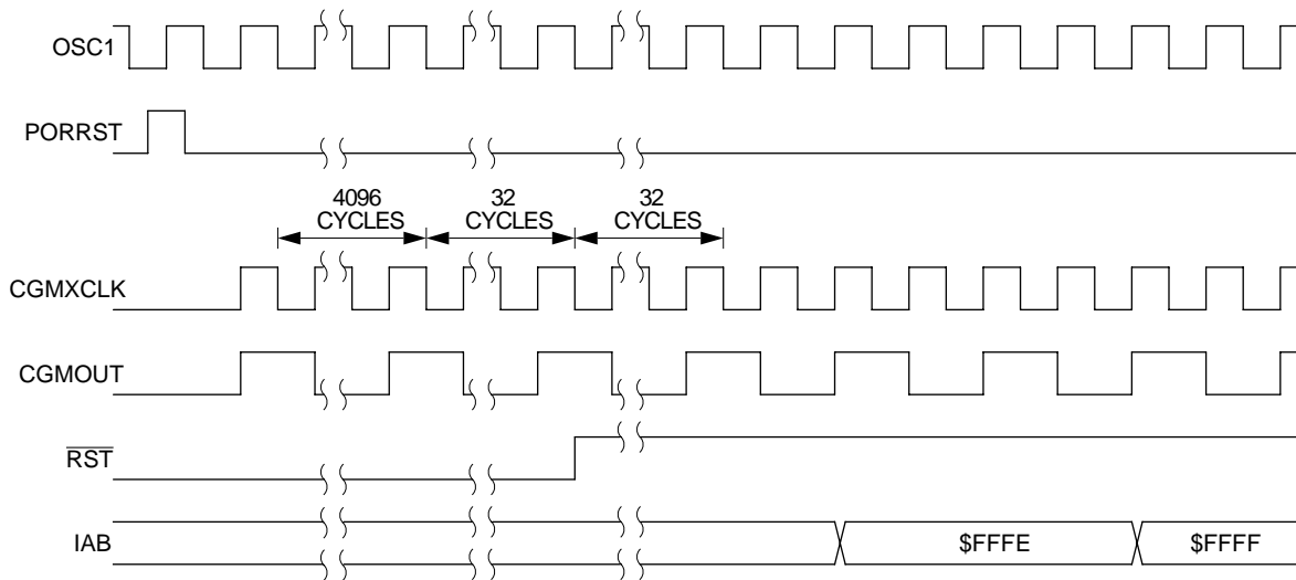
Figure 6. POR recovery
