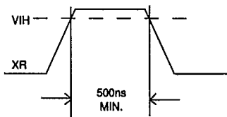
FIG. 9 XR PULSE
