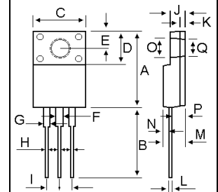
ITO-220
