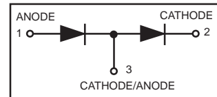
SOT-323 (SC-70)
