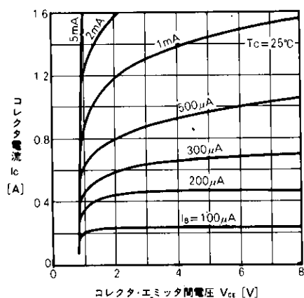
出力特性
