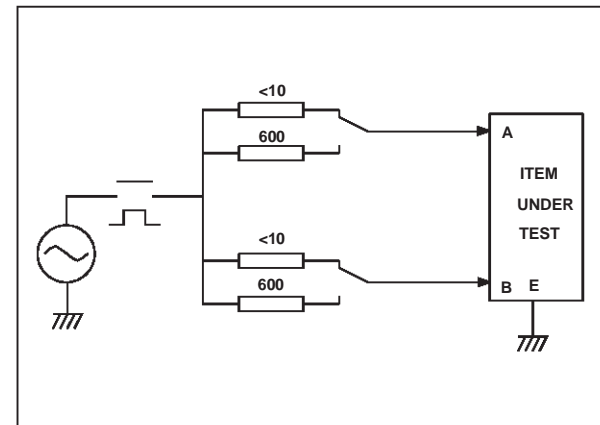
Fig. 12 : Power contact test circuit.
