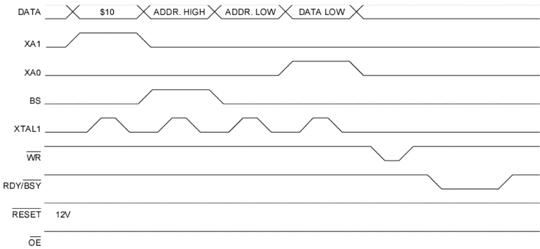
图 68 编程波形一
