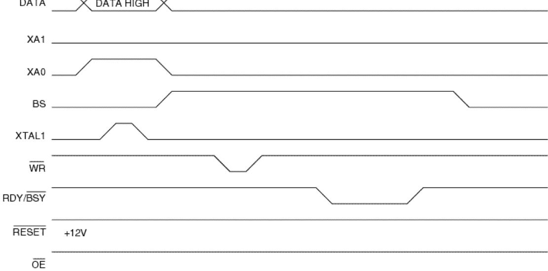
图 69 编程波形二
