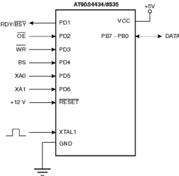
图 67 并行编程
