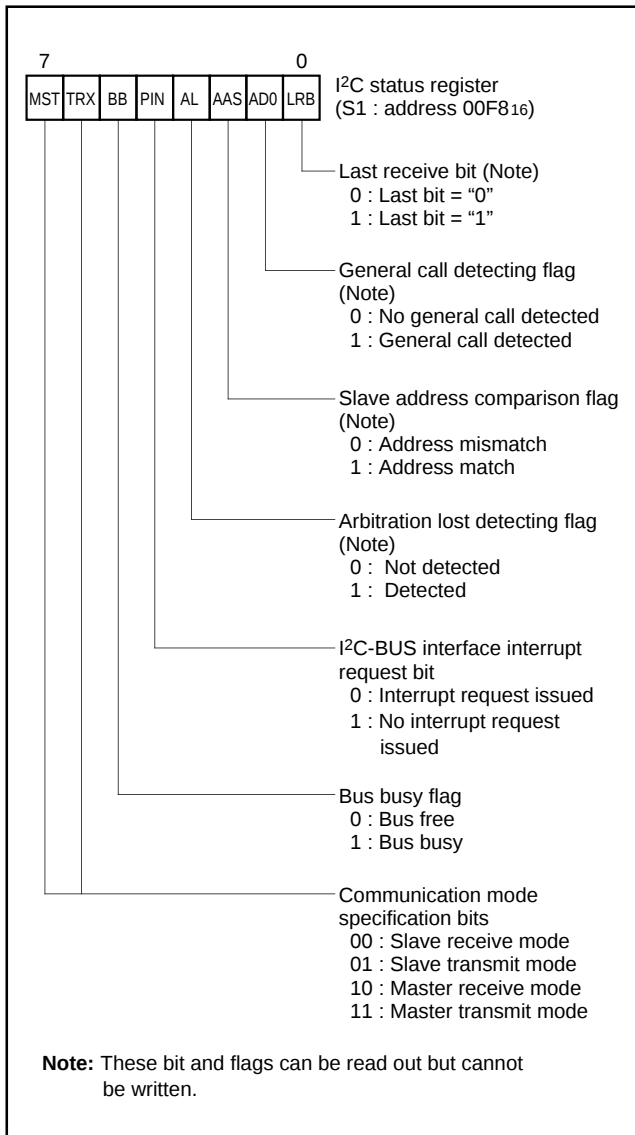
Fig. 39. I²C Status Register
