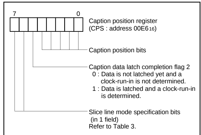
Fig. 28. Caption Position Register
