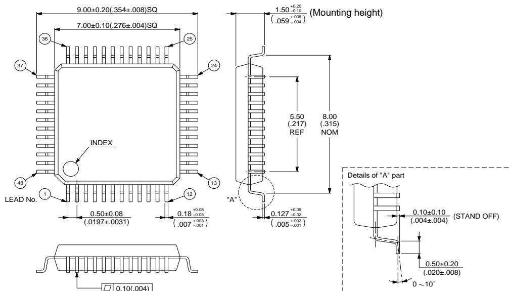
48 pin, Plastic LQFP (FPT-48P-M05)
