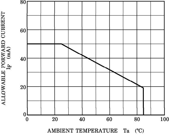
I_F - T_a
