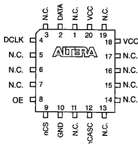
20-Pin PLCC
