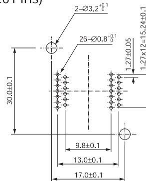
TSOP IC51-0442-1709 (44 Pins)
