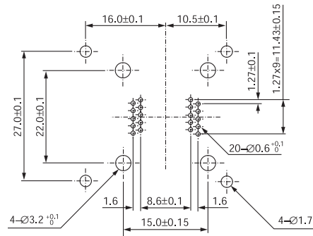
SOP IC51-0202-164 (20 Pins)
