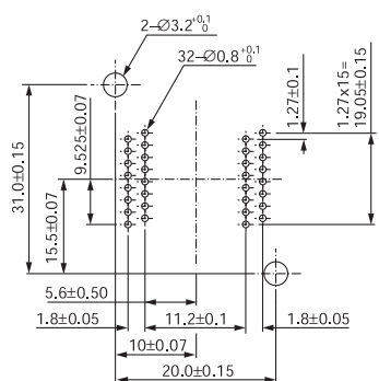
SOP IC51-0322-937 (32 Pins)
