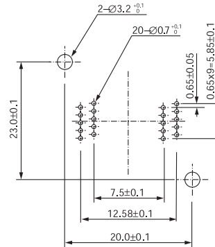
SSOP IC51-0202-912 (20 Pins)
