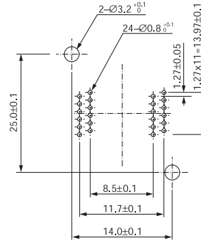
SOP IC51-0262-1339 (26 Pins)
