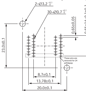
SSOP IC51-0302-755 (30 Pins)
