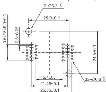
SSOP IC51-0322-910 (32 Pins)
