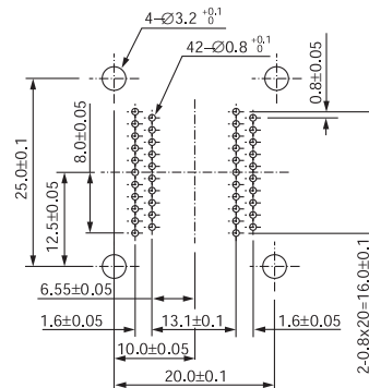
SOP IC51-0422-393 (42 Pins)
