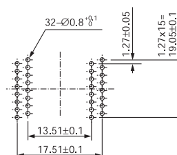
SOP IC51-0322-667-2 (32 Pins)
