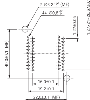
SOP IC51-0442-1315 (44 Pins)
