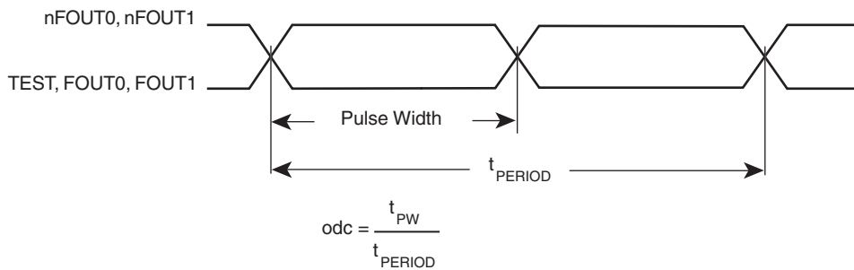
FIGURE 7 - odc & t_{PERIOD}
