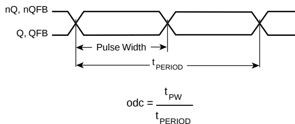
odc, t PW & t PERIOD
