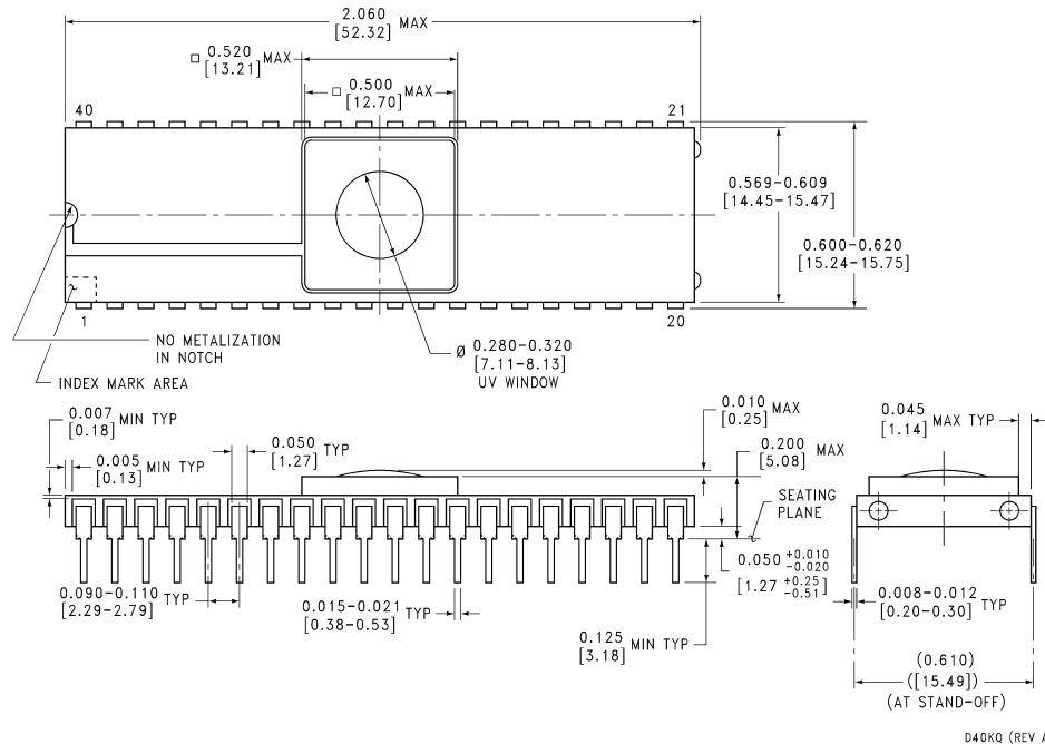
40-Lead Hermetic Dual-In-Line Package EPROM (D) Order Number COP8SGR740Q3 NS Package Number D40KQ
