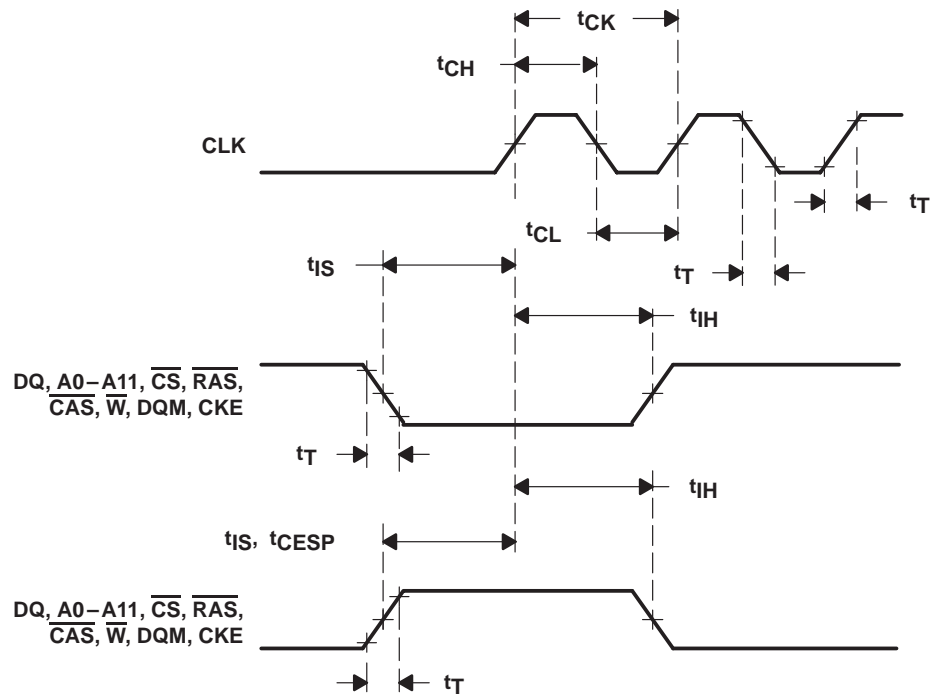
Figure 9. Input-Attribute Parameters
