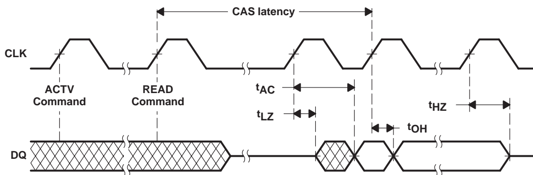
Figure 10. Output Parameters
